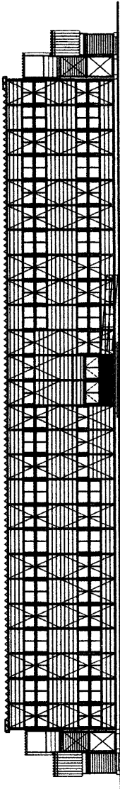
(113) 立面图 S=1:100
